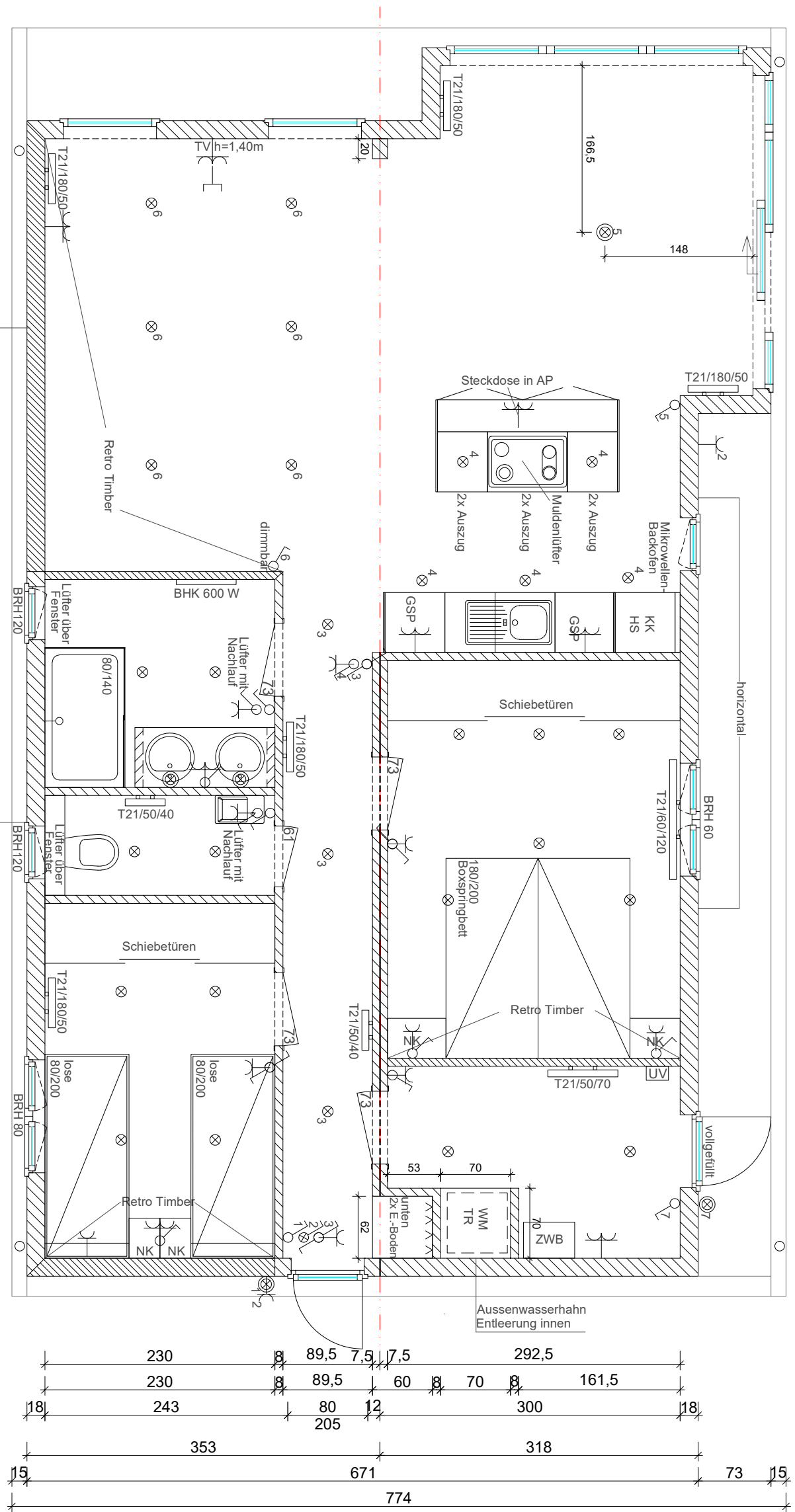
Ansicht B
